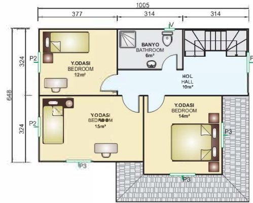
64 m 2 1. Kat Planı / First Floor Plan
