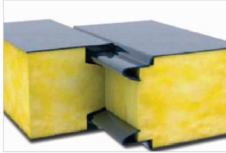
EPS, TAŞYÜNÜ ve CAMYÜNÜ PANELLERDE DİL VE OLUK
