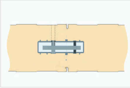
PUF PANELLERDE CAMLOCK BİRLEŞTİRME SİSTEMİ
